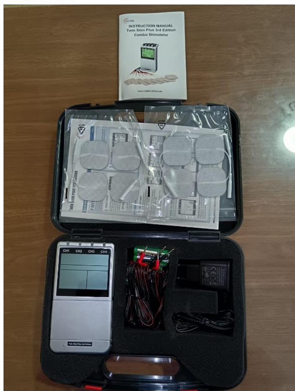
Simulatore elettrico di 4 canali
